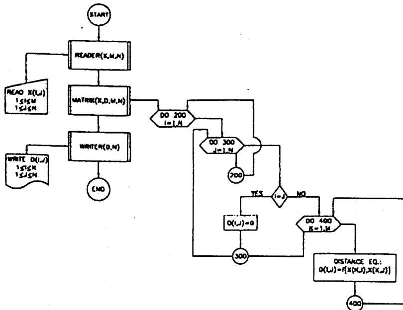
شکل ۱- نمودار جریان مربوط به تشکیل ماتریس R'
