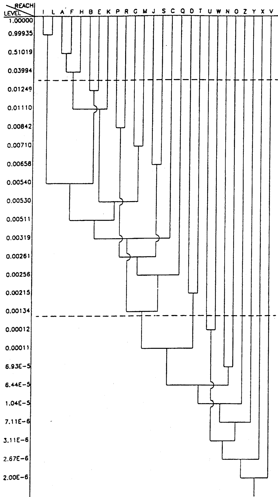
شکل ۷- نمودار درختی تحلیل کیفی رودخانه زاینده رود با فرض کنترل پارامترهای BOD، COD و EC - تابستان ۷۴
