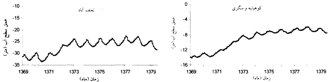
شکل ۶- نمودار سطح آب زیرزمینی در محدوده دشت نجف آباد و دشت کوهپایه و سگری تحت تأثیر سیاست پیشنهادی
