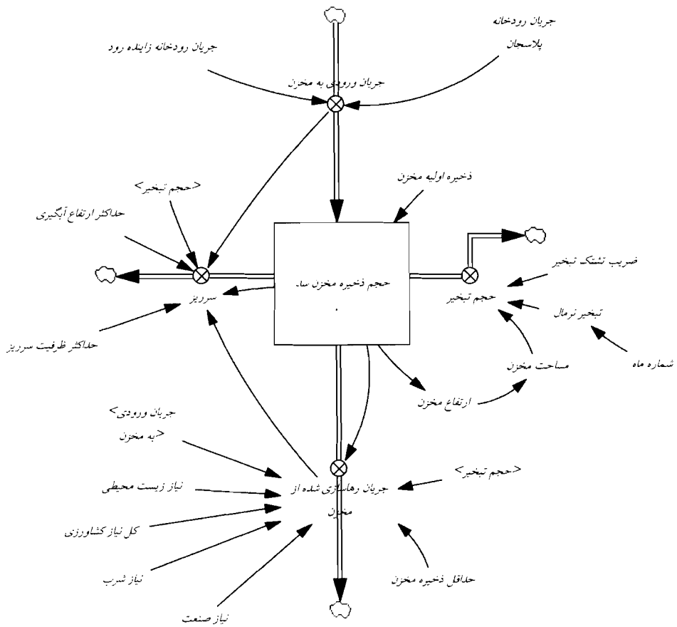
شکل ۱- قسمتی از مدل شامل مخزن سد، ورودی و خروجیها
